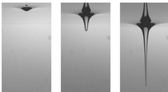
Slika 8. Fotografije vrtinca pri iztekanju iz okrogle vrteče se posode, iz [1].
