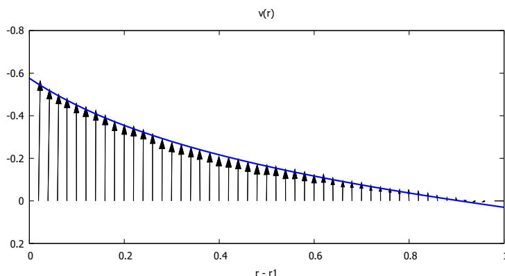
Slika 4. Radialna porazdelitev hitrosti pri toku med dvema valjema, dobljena s povprečenjem hitrosti ploščic pri danem radiju.
